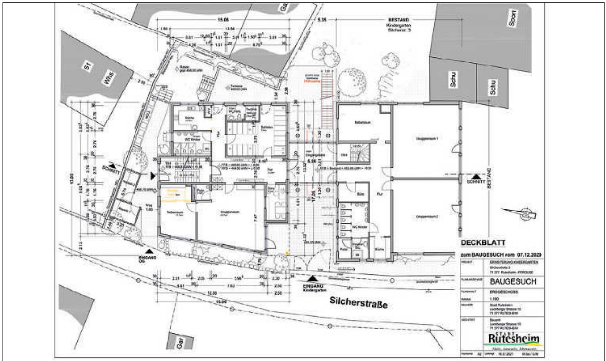
Grundriss Erdgeschoss
